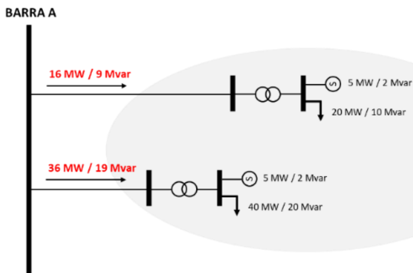
Figura 34 Sistema de potência a ser equivalentado - Geração
