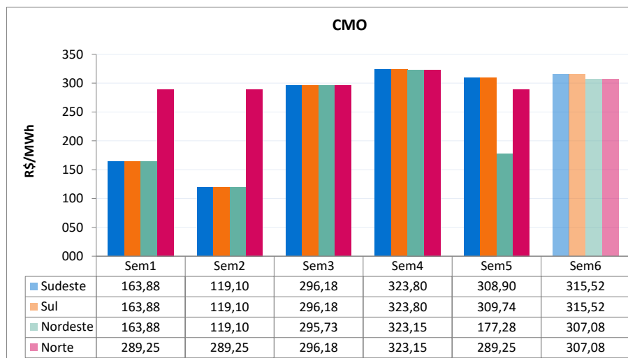
Figura 17 – CMO em valores médios
