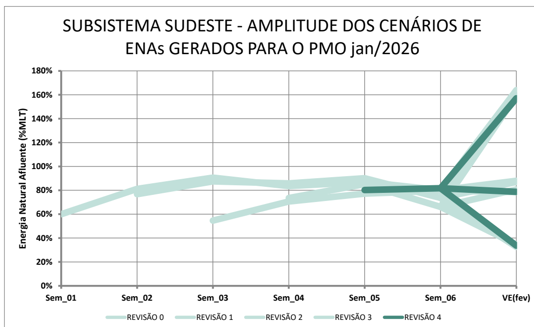
Figura 7 - Amplitude dos Cenários de ENA para o Subsistema Sudeste/Centro-Oeste, em %MLT, para a Revisão 4 de Janeiro/2026
