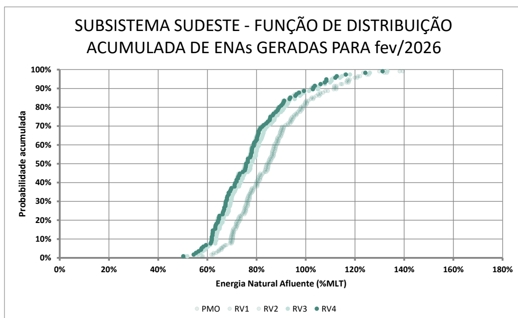
Figura 8 - Função de Distribuição Acumulada dos Cenários para o Subsistema Sudeste/Centro-Oeste para a Revisão 4 de Janeiro/2026
