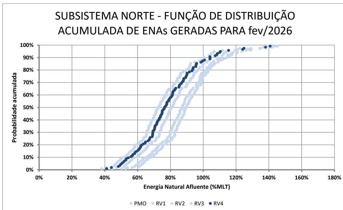
Figura 14 - Função de Distribuição Acumulada dos Cenários para o Subsistema Norte para a Revisão 4 de Janeiro/2026
