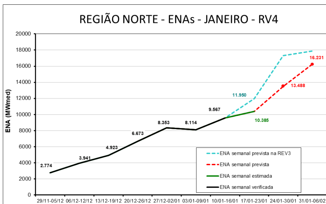
Figura 6 - Energias Naturais Afluentes ao Subsistema Norte das Revisões 3 e 4 do PMO de Janeiro/2026
