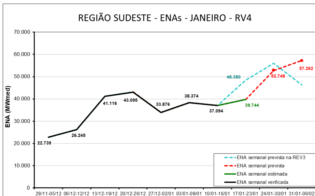
Figura 3 - Energias Naturais Afluentes ao Subsistema Sudeste/Centro-Oeste das Revisões 3 e 4 do PMO de Janeiro/2026
