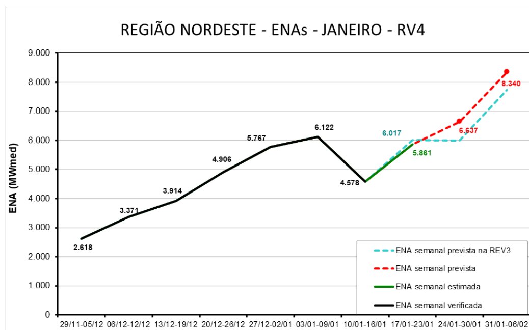
Figura 5 - Energias Naturais Afluentes ao Subsistema Nordeste das Revisões 3 e 4 do PMO de Janeiro/2026
