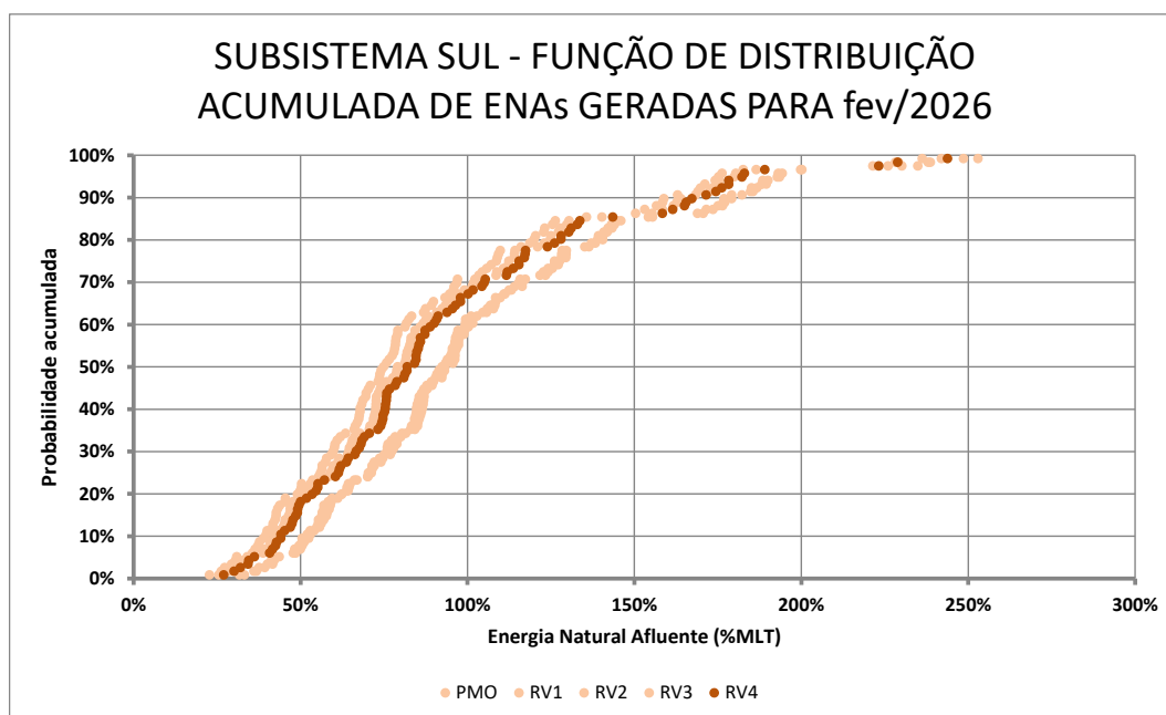
Figura 10 - Função de Distribuição Acumulada dos Cenários para o Subsistema Sul para a Revisão 4 de Janeiro/2026
