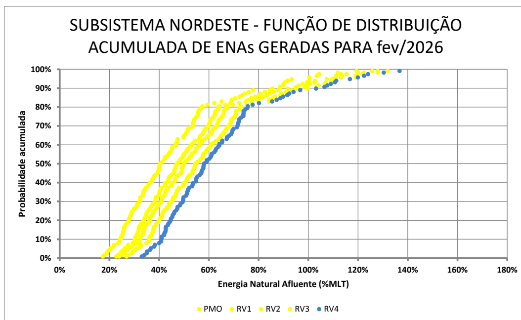
Figura 12 - Função de Distribuição Acumulada dos Cenários para o Subsystema Nordeste para a Revisão 4 de Janeiro/2026
