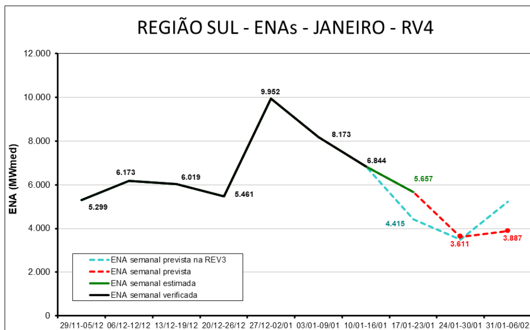
Figura 4 - Energias Naturais Afluentes ao Subsistema Sul das Revisões 3 e 4 do PMO de Janeiro/2026
