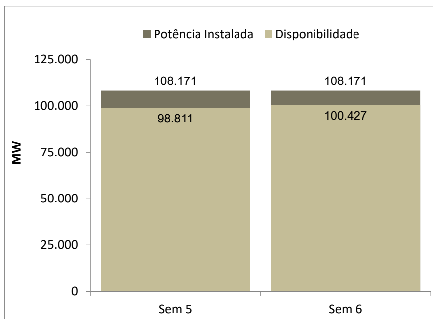
Figura 16 – Potência hidráulica disponível no SIN
