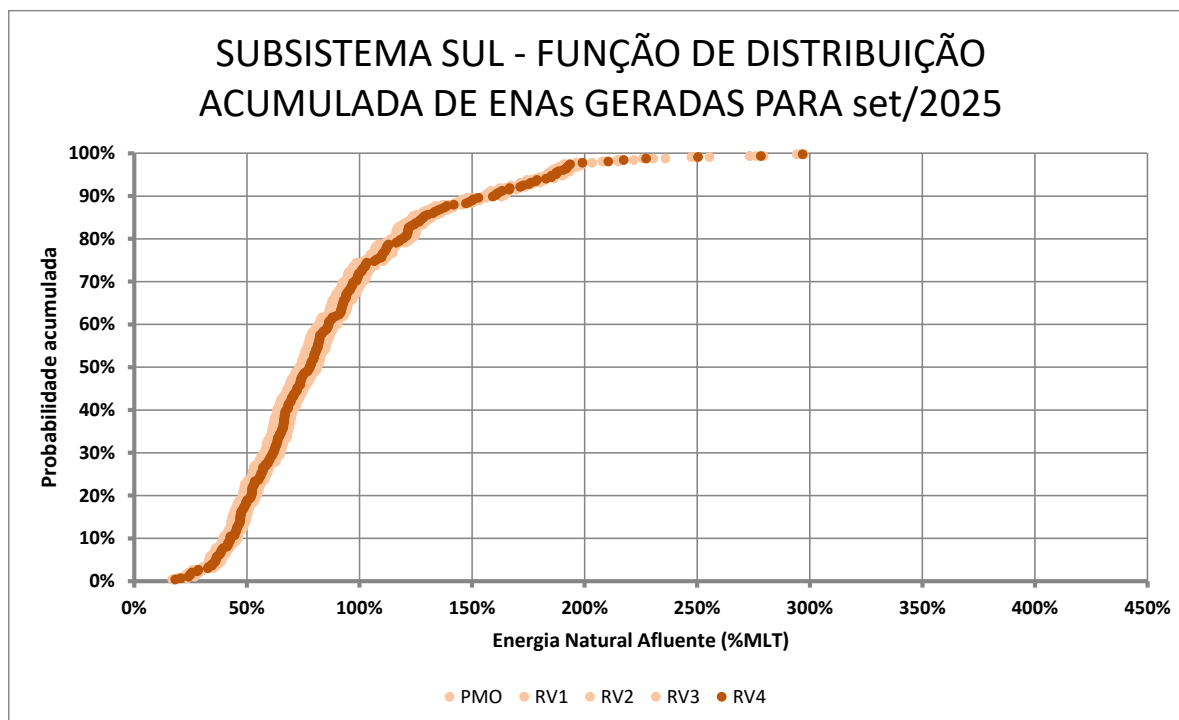
Figura 10 - Função de Distribuição Acumulada dos Cenários para o Subsystema Sul para a Revisão 4 de Agosto/2025
