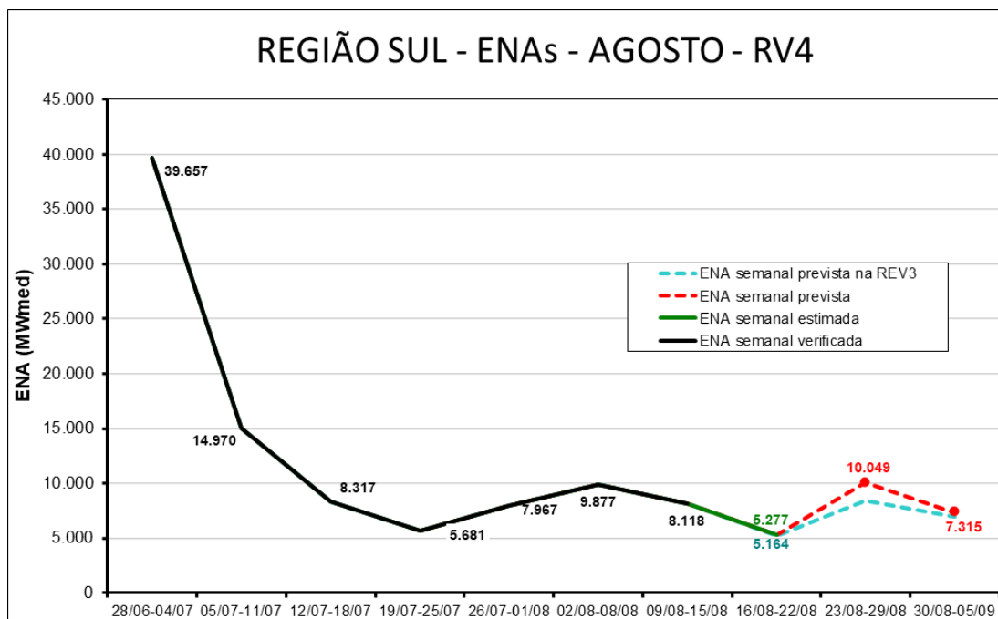
Figura 4 - Energias Naturais Afluentes ao Subsystema Sul das Revisões 3 e 4 do PMO de Agosto/2025
