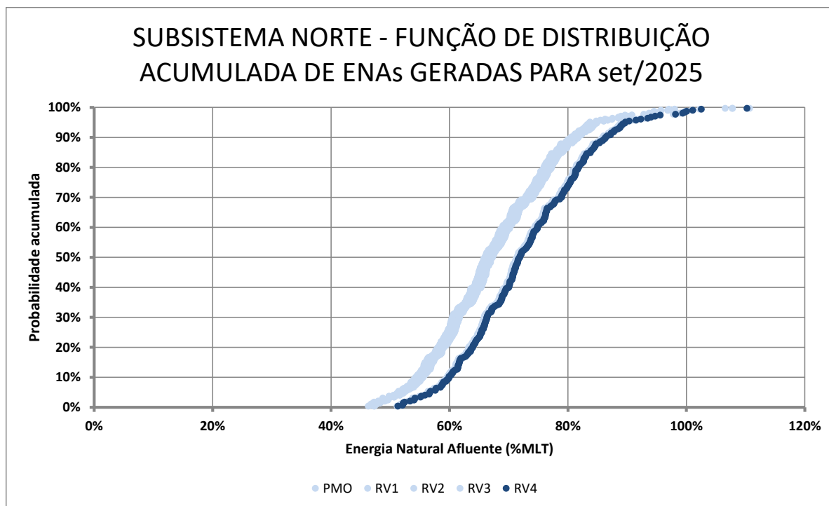
Figura 14 - Função de Distribuição Acumulada dos Cenários para o Subsistema Norte para a Revisão 4 de Agosto/2025
