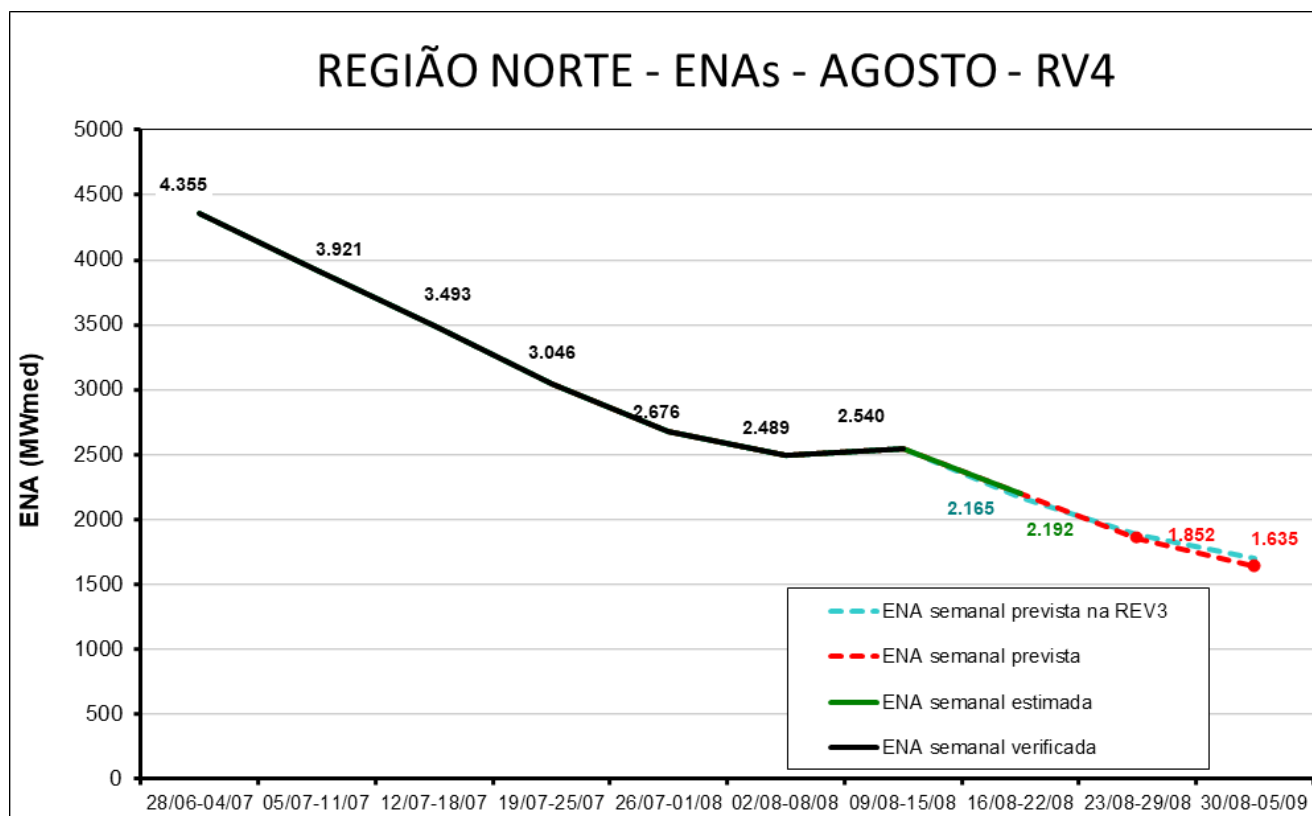
Figura 6 - Energias Naturais Afluentes ao Subsistema Norte das Revisões 3 e 4 do PMO de Agosto/2025
