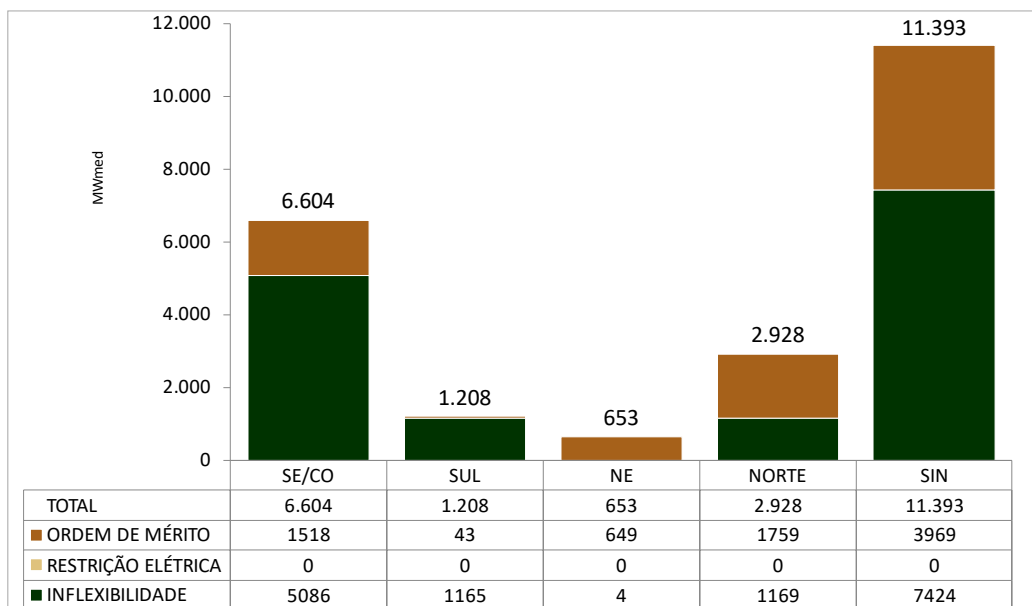
Figura 19 – Geração térmica para a próxima semana operativa
