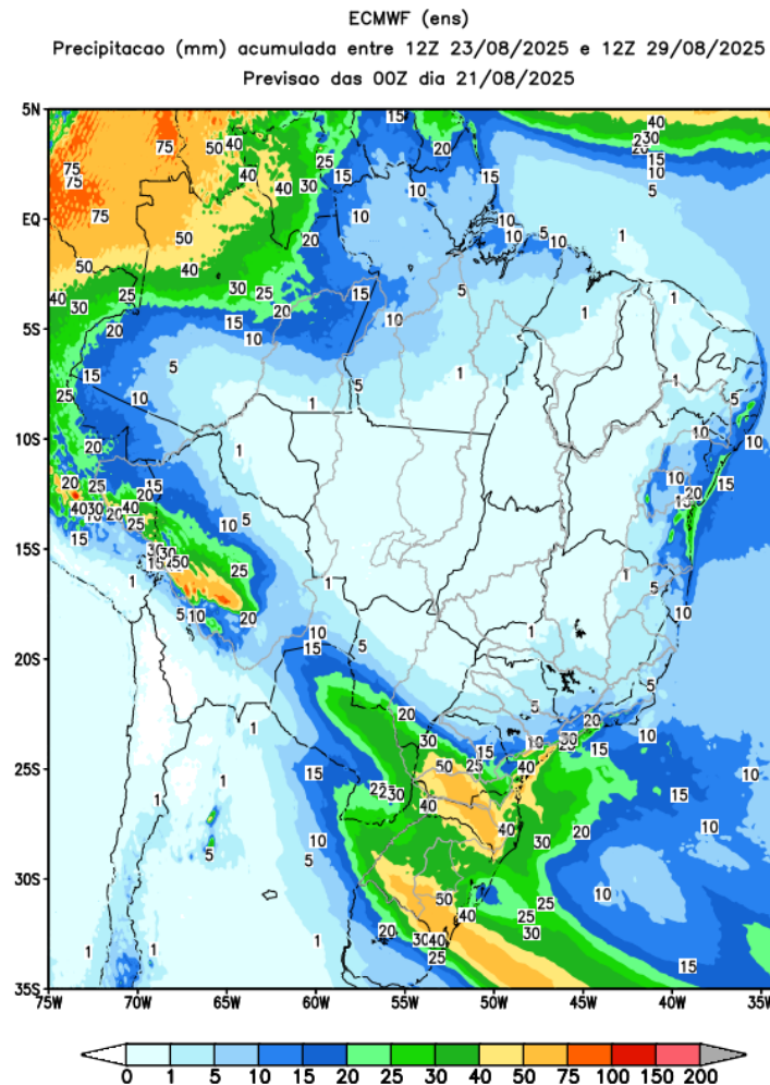
Figura 2 - Precipitação acumulada prevista pelo modelo ECMWF - período de 23 a 29/08/2025
