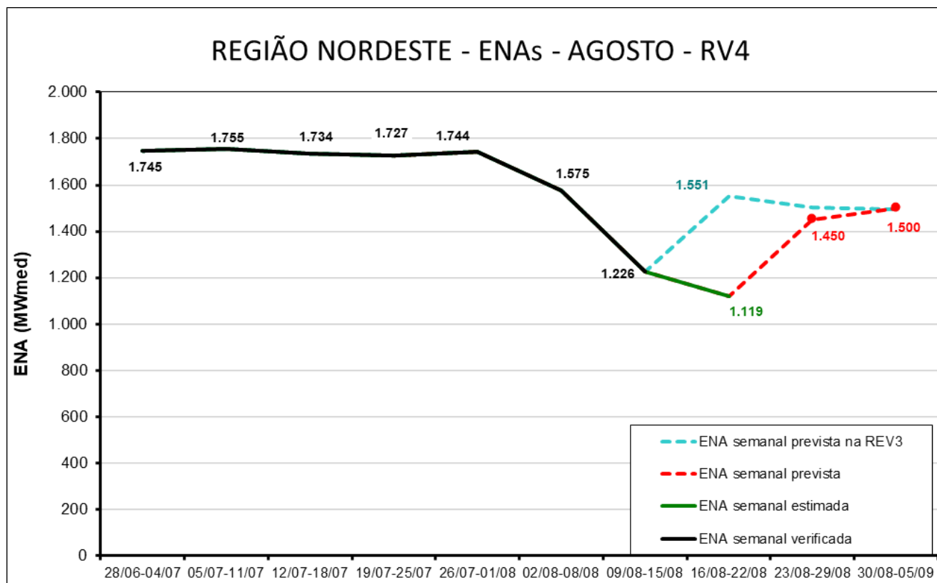
Figura 5 - Energias Naturais Afluentes ao Subsistema Nordeste das Revisões 3 e 4 do PMO de Agosto/2025
