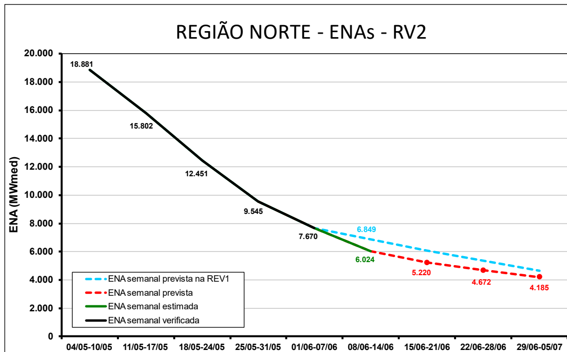
Figura 6 - Energias Naturais Afluentes ao Subsystema Norte das Revisões 1 e 2 do PMO de Junho/2024
