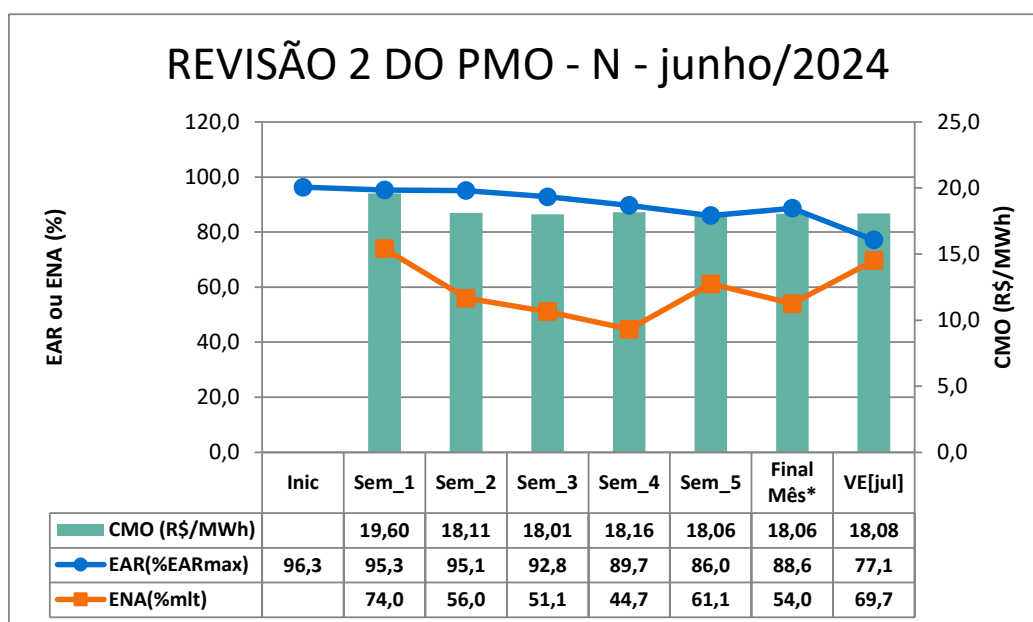
Figura 23 – Resumo de Junho/2024 para o Subsystema Norte
