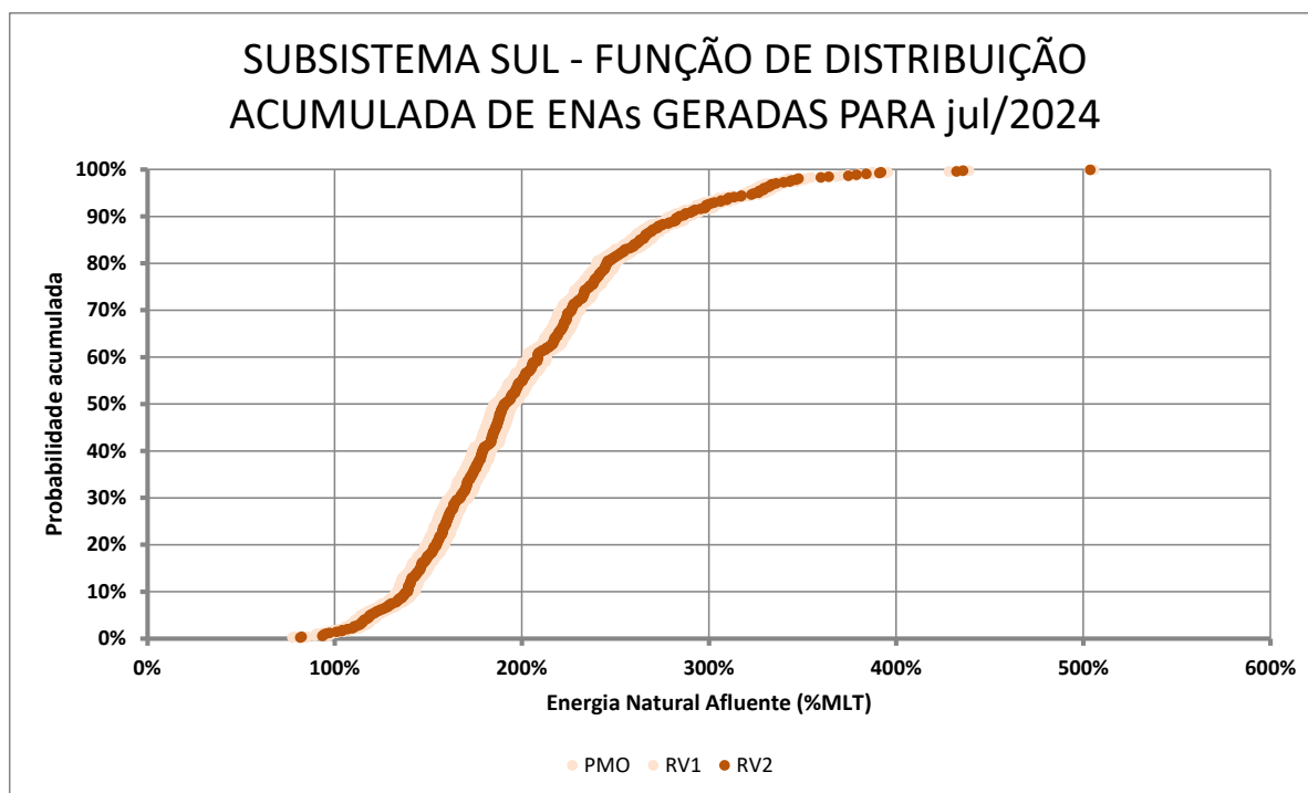
Figura 10 - Função de Distribuição Acumulada dos Cenários para o Subsystema Sul para a Revisão 2 de Junho/2024
