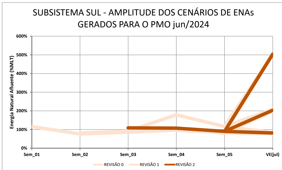
Figura 9 - Amplitude dos Cenários de ENA para o Subsystema Sul, em %MLT, para a Revisão 2 de Junho/2024
