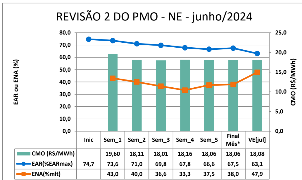
Figura 22 – Resumo de Junho/2024 para o Subsystema Nordeste
