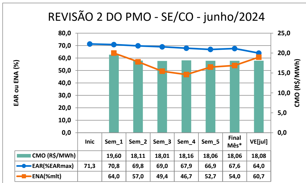
Figura 20 – Resumo de Junho/2024 para o Subsistema Sudeste/Centro-Oeste
