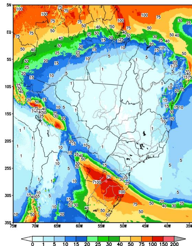
Figura 2 - Precipitação acumulada prevista pelo modelo ECMWF – 15 a 21/06/2024
