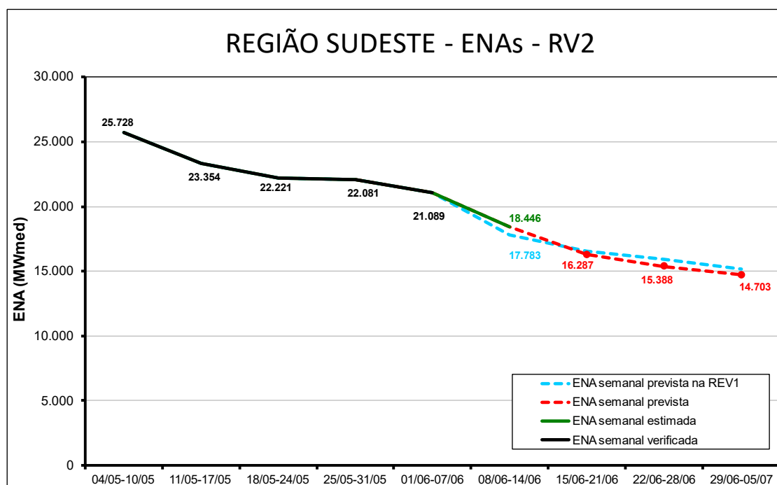
Figura 3 - Energias Naturais Afluentes ao Subsystema Sudeste/Centro-Oeste das Revisões 1 e 2 do PMO de Junho/2024
