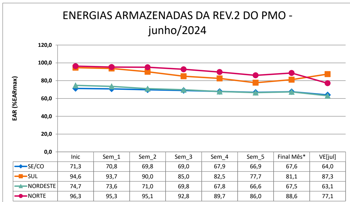
Figura 18 – Energias Armazenadas nas semanas operativas do mês de Junho/2024.
