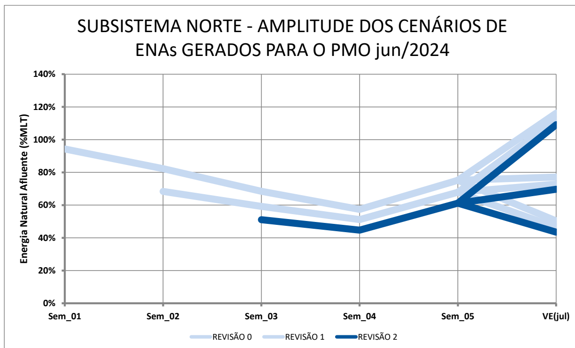
Figura 13 - Amplitude dos Cenários de ENA para o Subsistema Norte, em %MLT, para a Revisão 2 de Junho/2024
