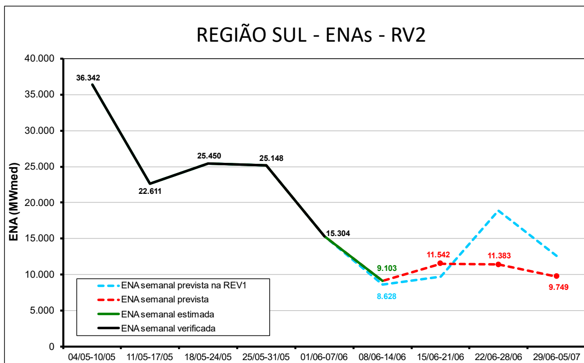
Figura 4 - Energias Naturais Afluentes ao Subsystema Sul das Revisões 1 e 2 do PMO de Junho/2024
