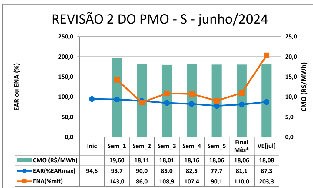
Figura 21 – Resumo de Junho/2024 para o Subsistema Sul
