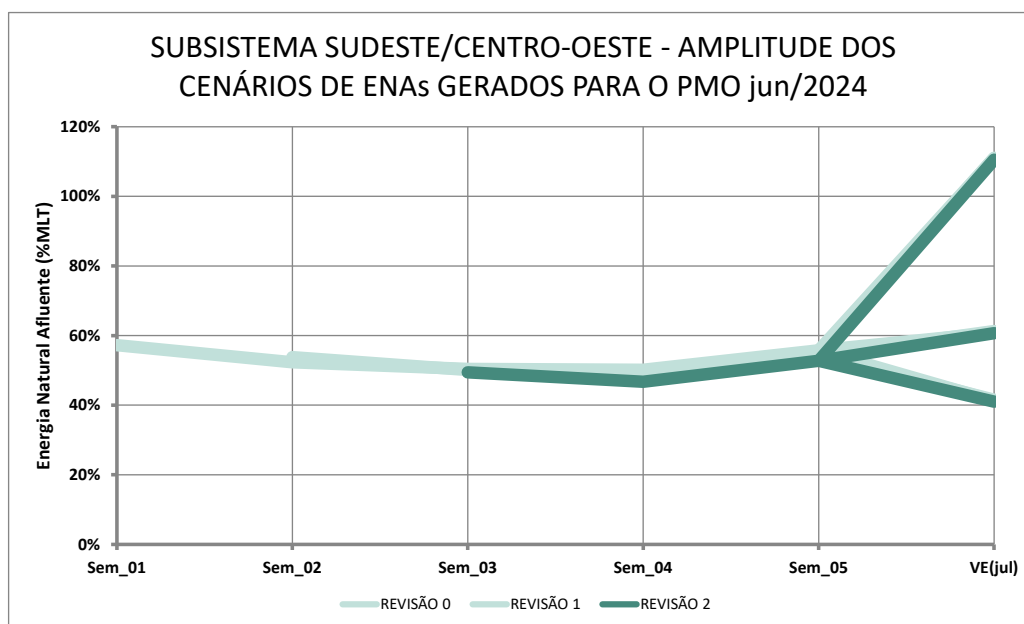
Figura 7 - Amplitude dos Cenários de ENA para o Subsistema Sudeste/Centro-Oeste, em %MLT, para a Revisão 2 de Junho/2024
