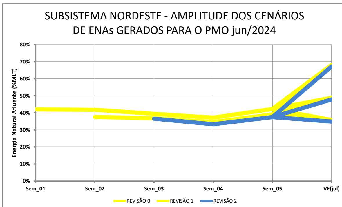
Figura 11 - Amplitude dos Cenários de ENA para o Subsystema Nordeste em %MLT, para a Revisão 2 de Junho/2024
