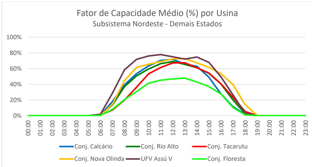
Figura 10 – Fator de capacidade médio no mês em base horária das usinas dos demais estados do subsistema Nordeste.
