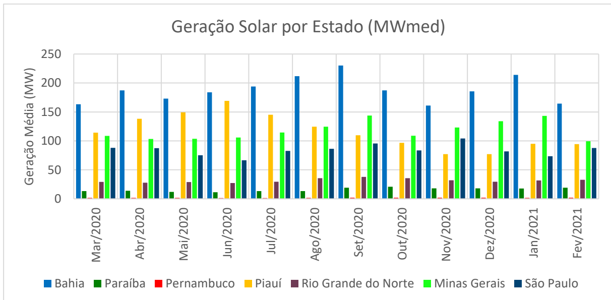
Figura 7 – Geração solar fotovoltaica média mensal (MWmed) nos últimos 12 meses por estado.
