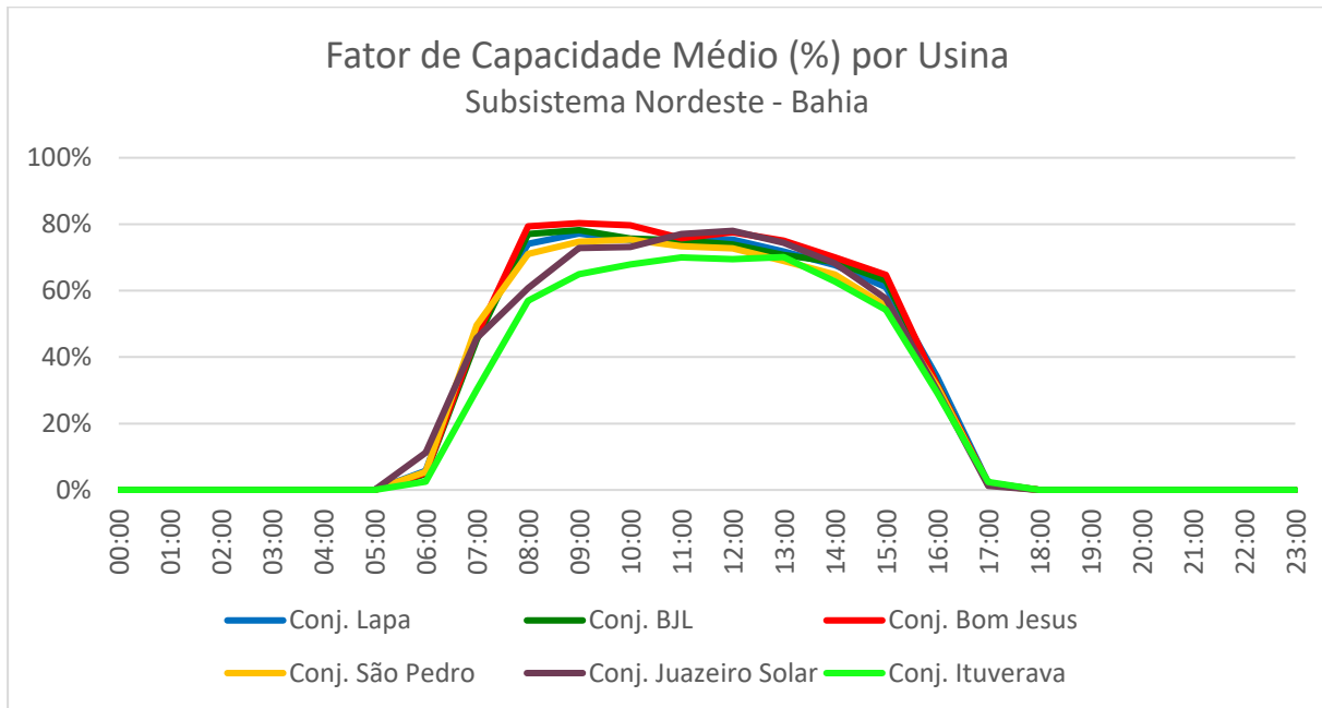
Figura 78 – Fator de capacidade médio no mês em base horária das usinas do estado da Bahia.
