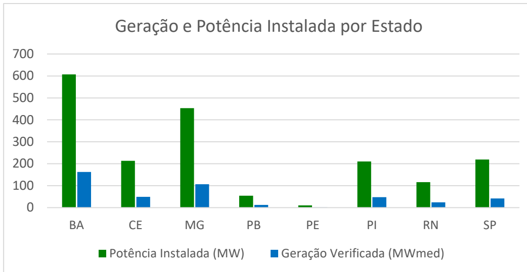
Figura 5 - Geração solar fotovoltaica média no mês por estado.
