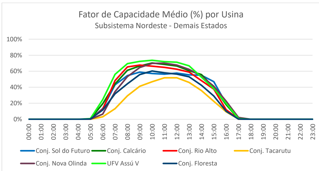
Figura 8 – Fator de capacidade médio no mês em base horária das usinas dos demais estados do subsistema Nordeste.
