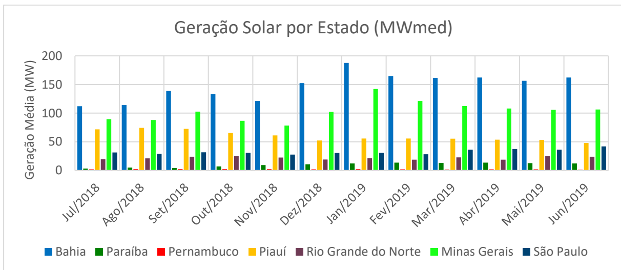
Figura 6 – Geração solar fotovoltaica média mensal (MWmed) nos últimos 12 meses por estado.
