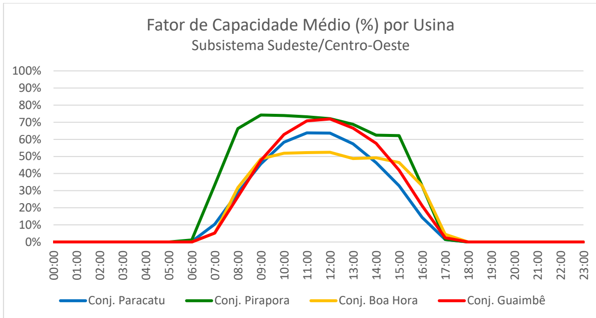
Figura 9 – Fator de capacidade médio no mês em base horária das usinas do subsistema Sudeste/Centro-Oeste.
