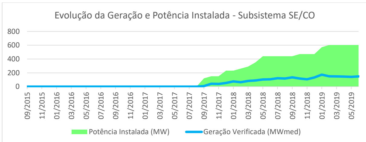
Figura 4 - Evolução da potência instalada de usinas solares fotovoltaicas e geração solar fotovoltaica verificada no Subsistema Sudeste/Centro-Oeste. As primeiras usinas entraram em operação no mês de setembro de 2017, totalizando 120 MW.
