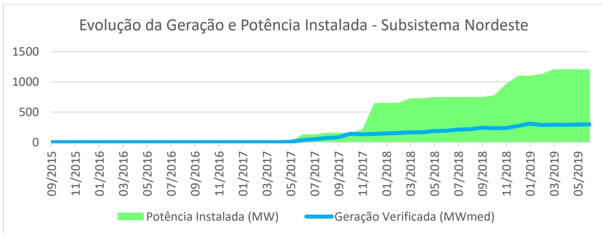
Figura 3 - Evolução da potência instalada de usinas solares fotovoltaicas e geração solar fotovoltaica verificada no Subsistema Nordeste. As primeiras usinas entraram em operação no mês de setembro de 2015, totalizando 10 MW.
