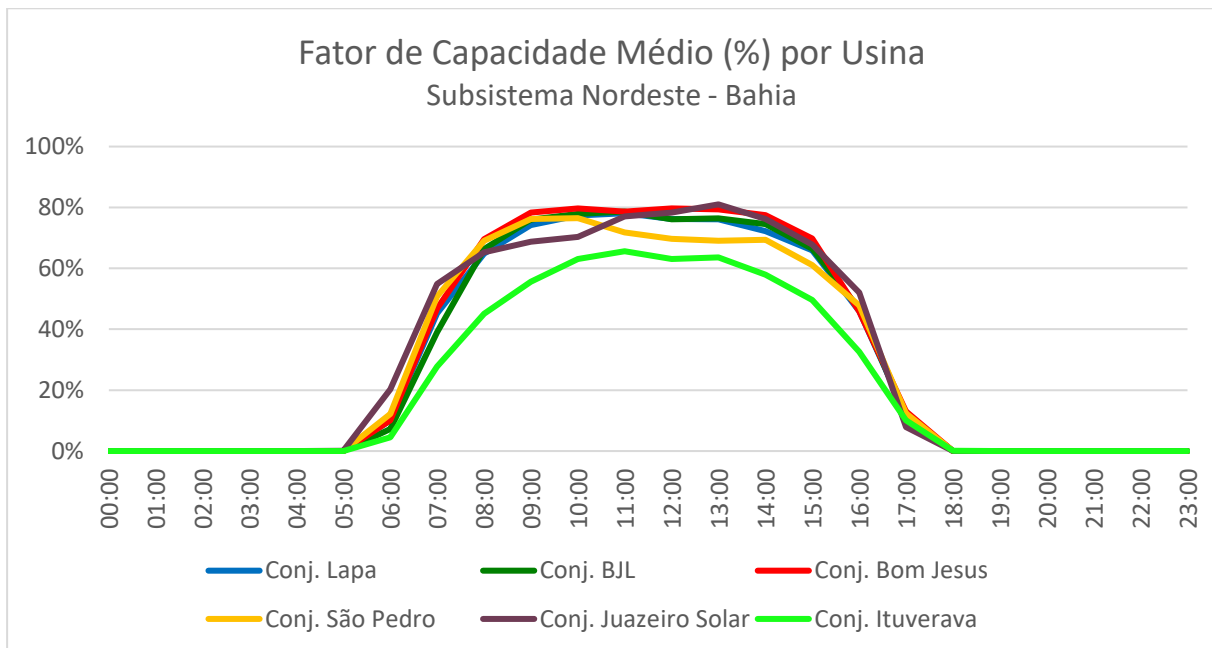
Figura 98 – Fator de capacidade médio no mês em base horária das usinas do estado da Bahia.
