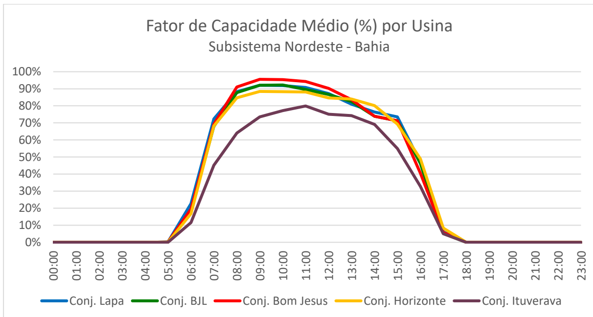
Figura 498 – Fator de capacidade médio no mês em base horária das usinas do estado da Bahia.
